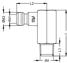
Plugs / Nippel
