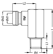
Plugs / Nippel
