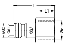
Plugs / Nippel
